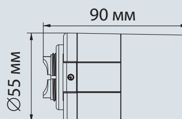
З адаптером для клапана Giacomini
